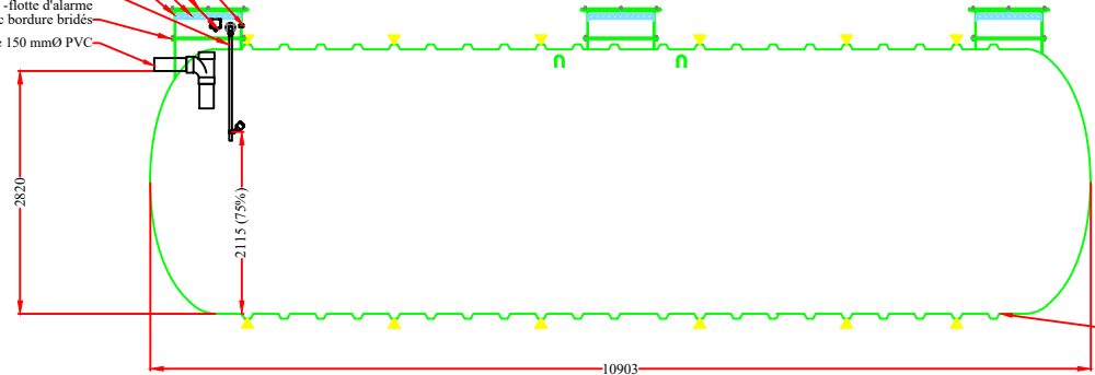
Z100SW-75000FV préfabriqué, préassemblé de MEi Assainissement
